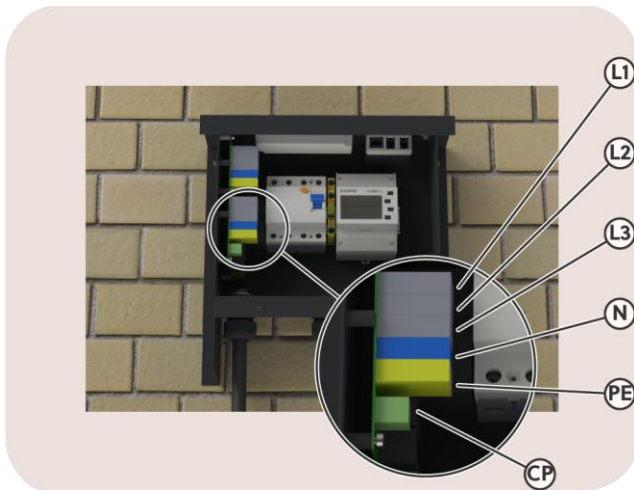
Abbildung 10: Blick auf die Kabelverbindungen
