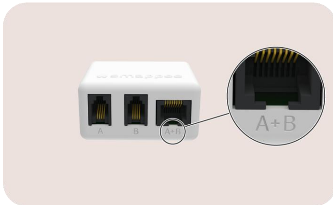
Abbildung 13: Blick auf die A+B-Anschlüsse des Smappee Splitters
