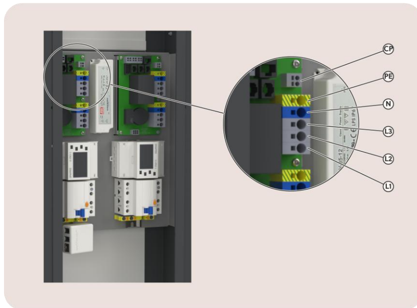
Abbildung 10: Blick auf die Kabelverbindungen
