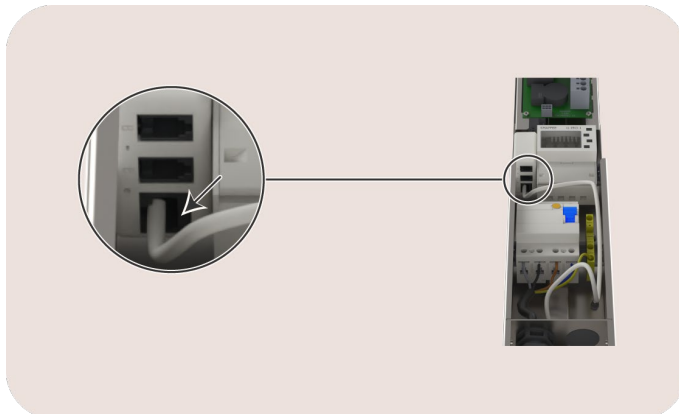
Afbeelding 18: aanzicht op de Smappee Connect
