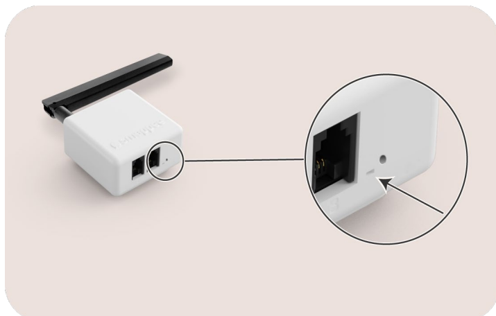
Afbeelding 33: positie van de led op de Smappee 4G Connect (antenne niet weergegeven)
