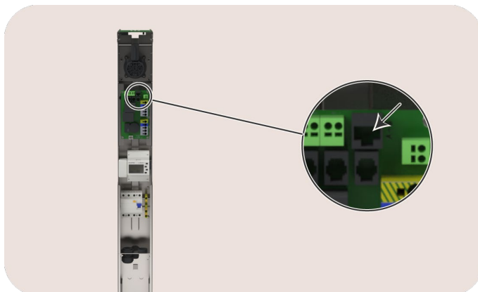
Afbeelding24: aanzicht op de A+B-poort van het relaisbord
