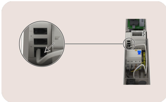
Afbeelding17: zicht op de RJ45-poort
