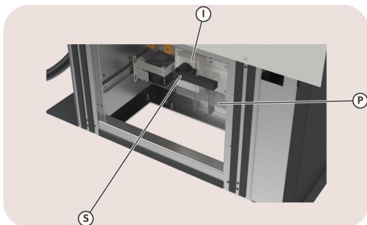
Abbildung 26: Blick auf den Lastschutzschalter
