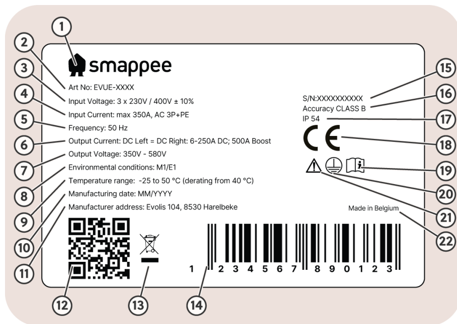
Abbildung 3: Position des Typenschildes
