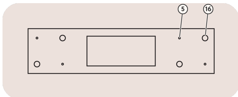
Afbeelding 8: Bovenaanzicht van de gaten in de vloerplaat
