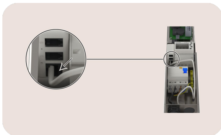
Image 17 : Vue sur le port RJ45
