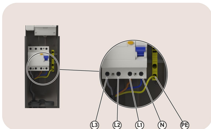
Image 15 : Vue sur la connexion de l'alimentation électrique
