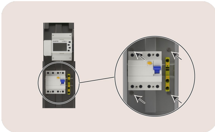
Abbildung 9: Ansicht der Rückseite der EV One
