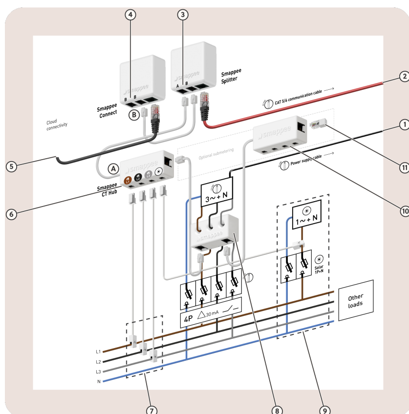
Image 27 : Schéma de connexion 3 x 400 V + N
