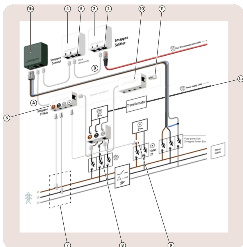
Image 26 : Schéma de connexion 3 x 230 V - avec transformateur
