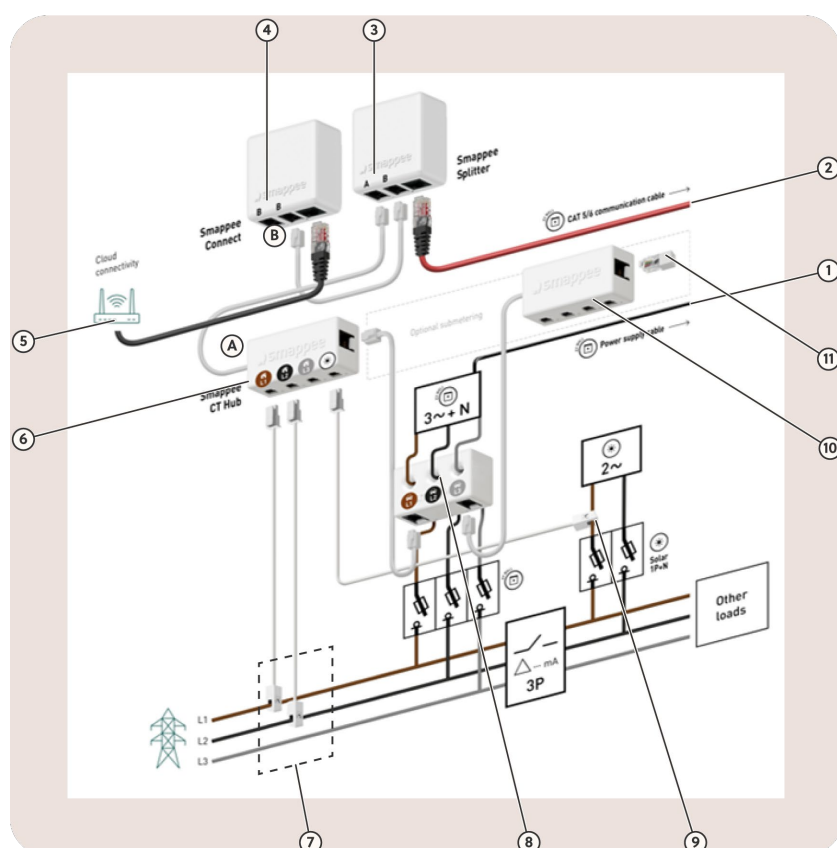
Image 25 : Schéma de connexion 3 x 230 V - sans transformateur
