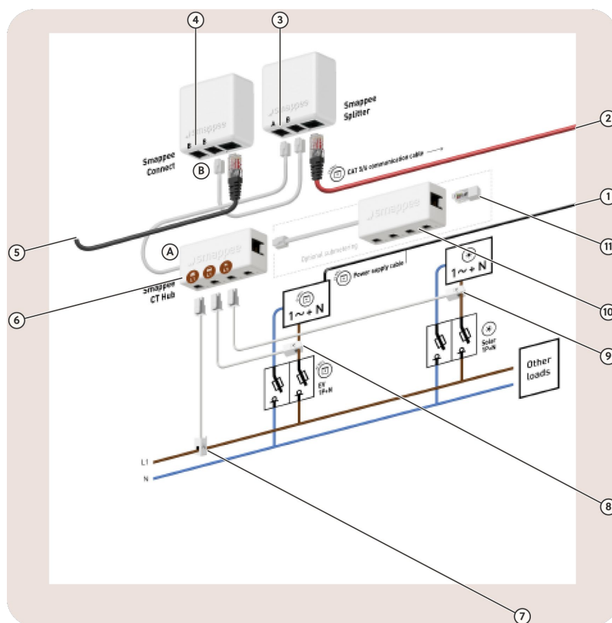
Image 19 : Schéma de connectivité 1 X 230 V + N
