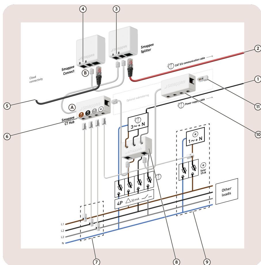
Image 22 : Schéma de connectivité 3 x 400 V + N
