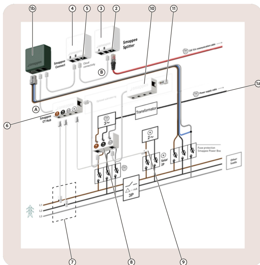
Image 21 : Schéma de connectivité 3 x 230 V - avec transformateur
