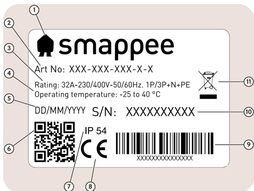
Image 4 : Étiquette d'identification
