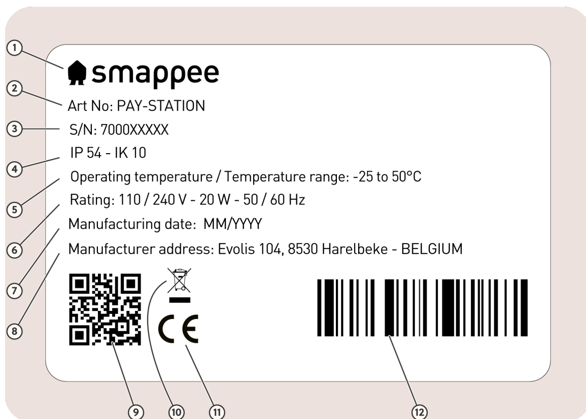
Afbeelding 3: identificatielabel
